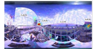
γイメージャーによる測定結果例 (原子炉建屋等の外観)
