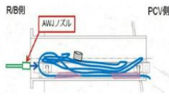
堆積物除去装置 (高圧水、AWJ) ※遠隔作業 ドーザツールによる堆積物の押し込み、 高圧水・AWJの噴射による堆積物の除去
