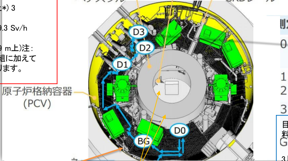
圧力容器の土台(ペDESTAL)・開口部 ペDESTAL CRDレール
