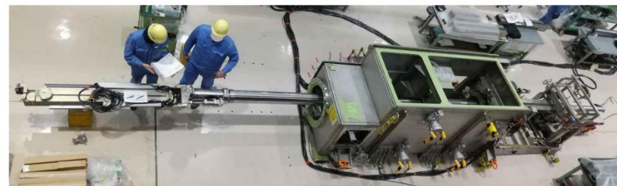
テレスコ式試験的取り出し装置 (装置を上方から撮影)
