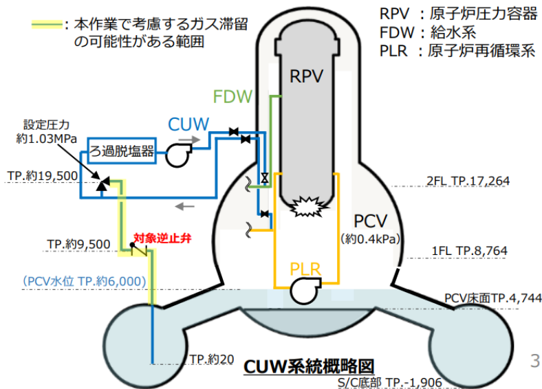
(CUW系統概略図)
