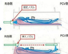
堆積物除去 (低圧水) ※遠隔作業 ドーザツールによる堆積物の押し込み、 低圧水の噴射による堆積物の除去
