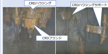
CRD関連機器の状況(左：ハウジング、右：サポート)
