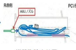
堆積物除去装置 (高圧水、AWJ) ※遠隔作業 ドーザツールによる堆積物の押し込み、 高圧水・AWJの噴射による堆積物の除去
