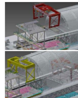
カーダ上吊り込みイメージ
