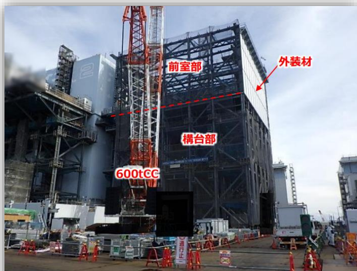
現場全景[南西側] (撮影日: 2024.2.9)
