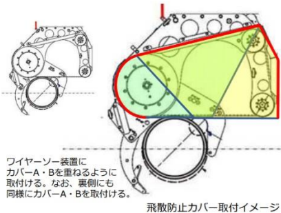
飛散防止カバー取り付けイメージ
