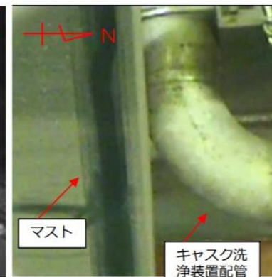
マストとの干渉の状況(No.⑭※)
