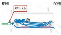
堆積物除去装置 (高圧水、AWJ)
