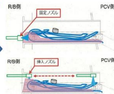
堆積物除去 (低圧水) ※遠隔作業 ドーザツールによる堆積物の押し込み、 低圧水の噴射による堆積物の除去
