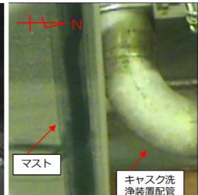
マストとの干渉の状況(No.⑭※)
