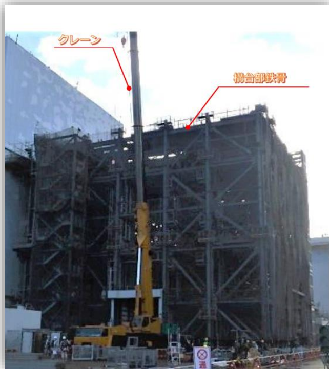
(組み立てが完了した構台の鉄骨ユニット)
